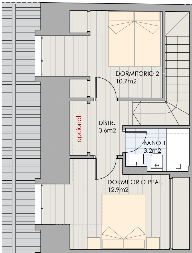
PLANTA BAJOCUBIERTA
